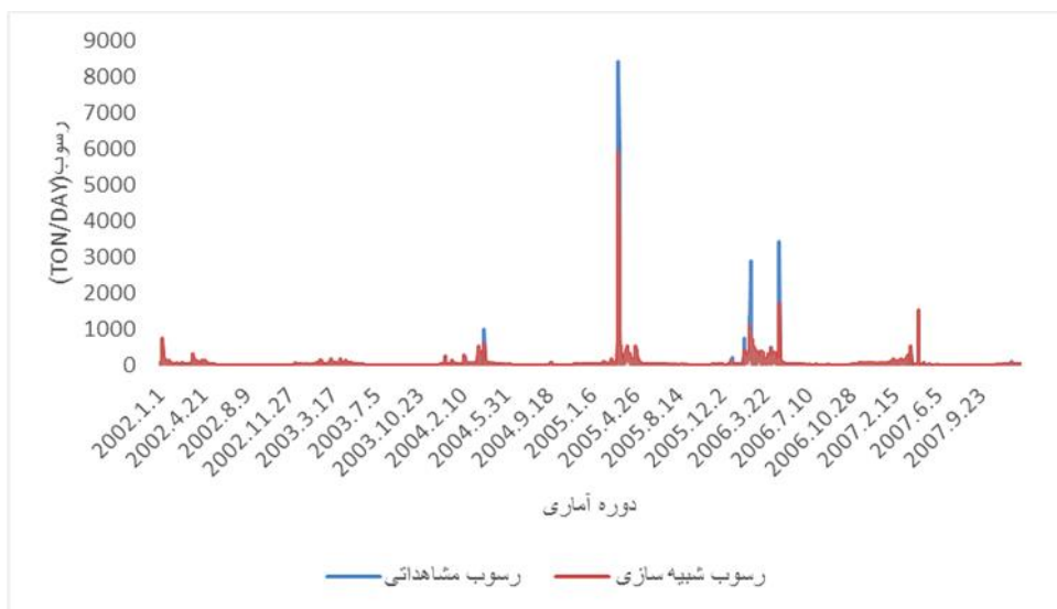
شکل ۴- رسوب متناظر شبیه‌سازی و مشاهده‌ای دوره واسنجی 2002-2007 Figure 4. Observed and simulated daily sediment Calibration period (2002-2007)
