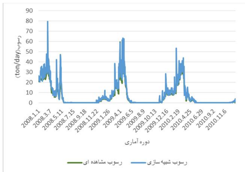
شکل ۵- رسوب متناظر شبیه‌سازی و مشاهده‌ای روزانه، دوره اعتبارسنجی ۲۰۰۸-۲۰۱۰ Figure 5. Simulated and Observed values of daily sediment Validation period (2010-2008)
