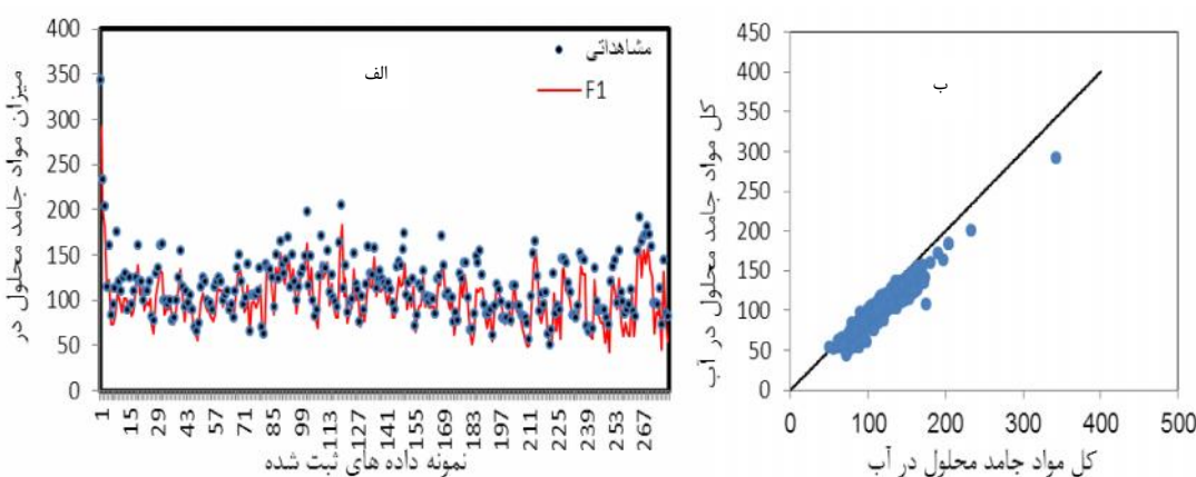
شکل ۵- نمودار حاصل از مقادیر بهینه مدل برنامه‌ریزی بیان ژن برای داده‌های ثبت‌شده مرحله صحت سنجی (الف) مقادیر محاسباتی و مشاهداتی نسبت به زمان (ب) نمودار پراکنش میان مقادیر مشاهداتی و محاسباتی Figure 5. Diagram of optimal values of gene expression programming model for recorded data in validation phase A) the observed and computed values over time B) scattered plot of observed and computed values
