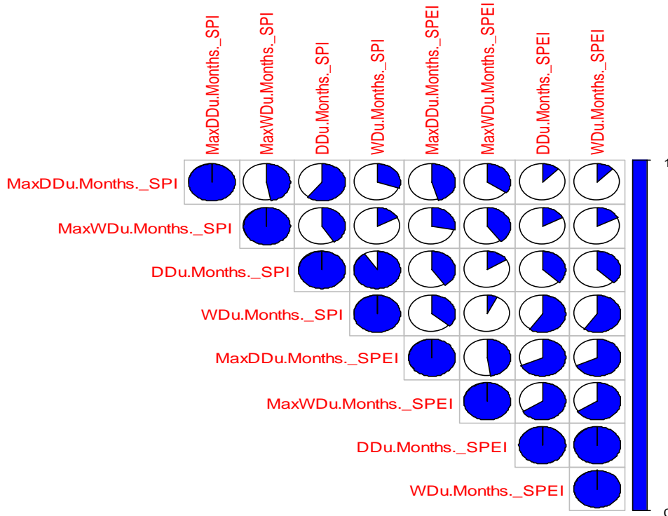
شکل ۸- همبستگی بین شاخص‌های SPI و SPEI در تعیین تعداد ماه‌های ترسالی و خشکسالی Figure 8. Correlation of SPI and SPEI indices in determining the number of wet and dry spells months
