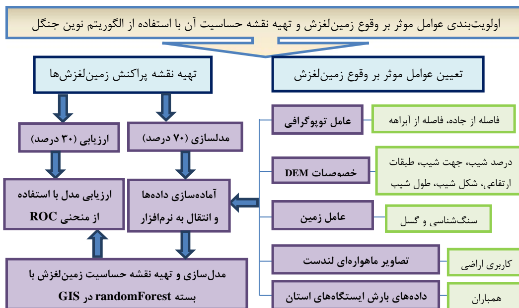
شکل ۲- نمودار جریان‌ی تهیه نقشه حساسیت زمین لغزش با استفاده از الگوریتم جنگل تصادفی Figure 2. Flowchart of landslide susceptibility mapping using random forest algorithm
