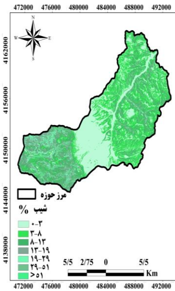
شکل ۵- نقشه شیب حوزه آبخیز روضه‌چای
