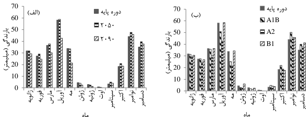
شکل ۵- الف: مقایسه بارندگی ماهانه ایستگاه میاندواب بر اساس سناریو A2 در سه دوره. ب: مقایسه بارندگی ماهانه ایستگاه میاندواب در دوره پایه و دوره ۲۰۹۰ بر اساس سناریوهای A1B، A2 و B1 Figure 5. a: Comparison of the monthly precipitation in Miandoab station based on scenario A2 in three periods. b: Comparison of the monthly precipitation in Miandoab station in the base period and 2090 based on three scenarios A1B, A2 and B1
